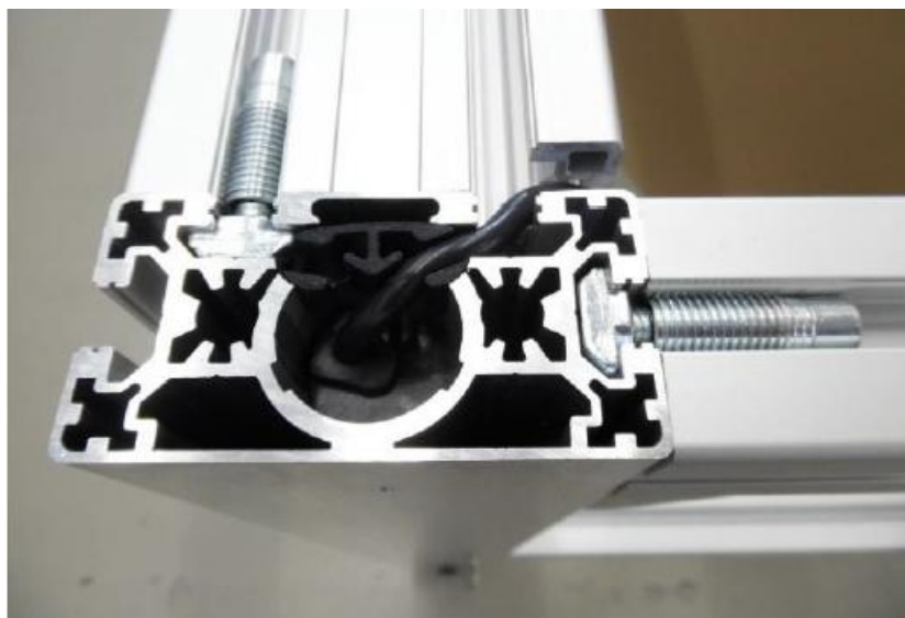
Abbildung 12: SMS-B-45x90: Beispiel zur Verbindung Hubelement mit Grundrahmen mittels handelsüblicher Bolzenklemmverbinder
