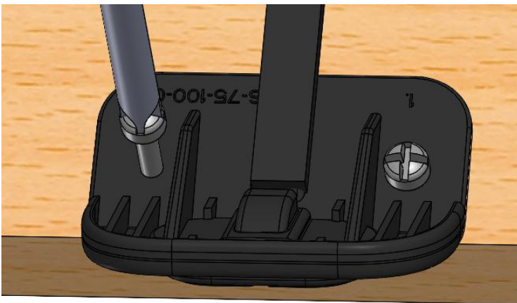
Abbildung 20: Befestigung UP / Down Handschalter LM2LCDP
