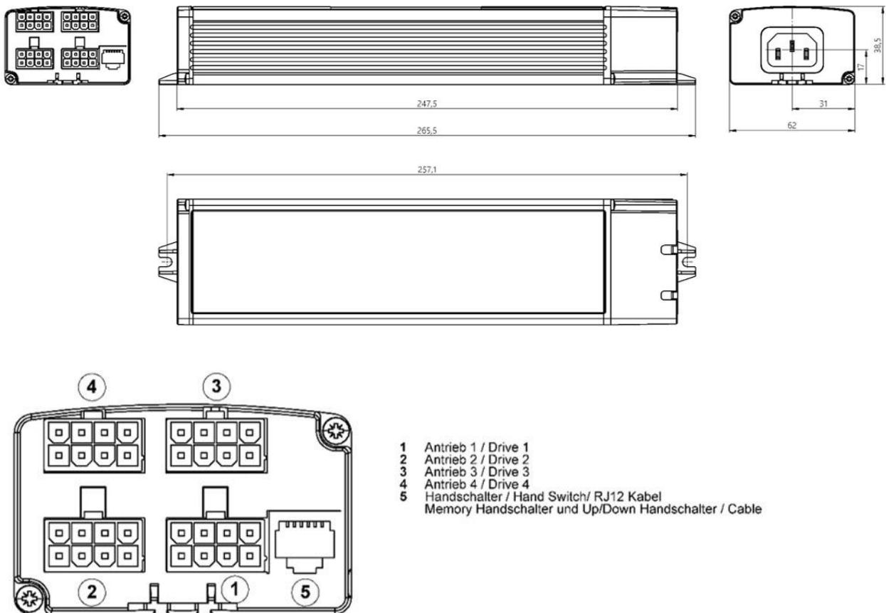
Abbildung 17: Elektrische Steuerung Abmessungen-Anschlüsse
