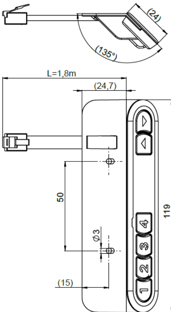
Abbildung 23: Abmaße des Memory Handschalters LD6LC
