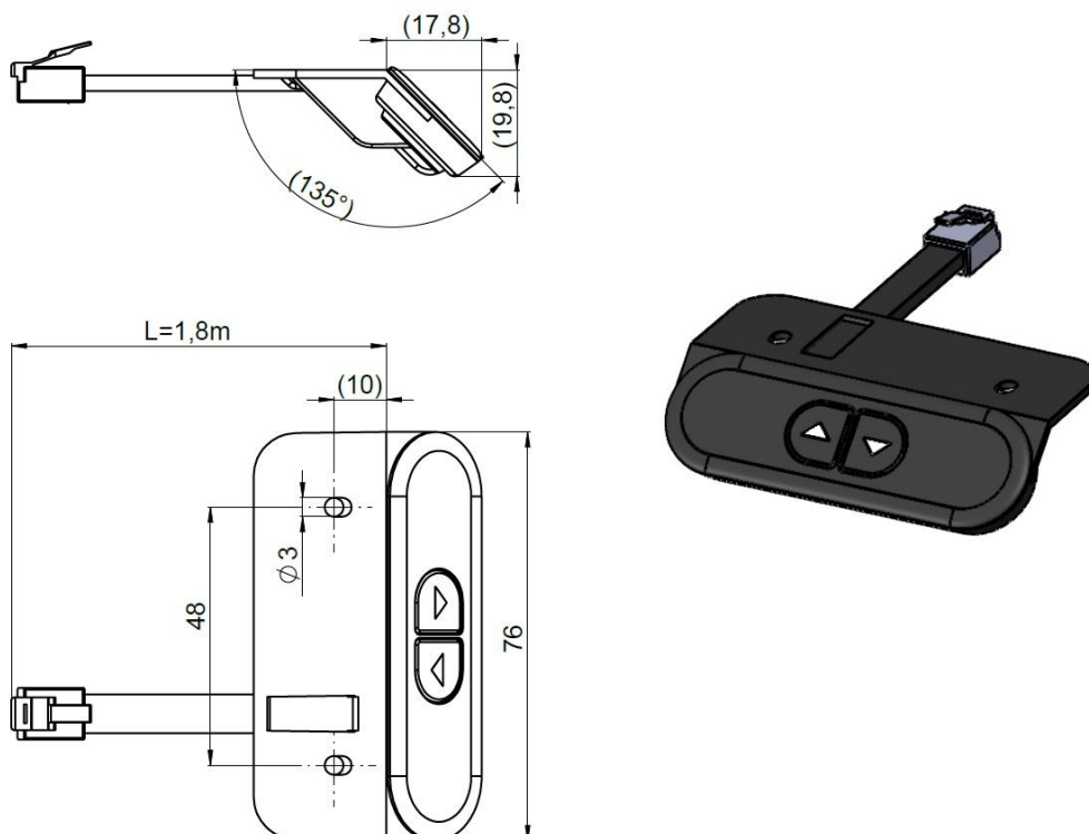
Abbildung 21: Abmaße UP / Down Handschalter LM2LCDP
