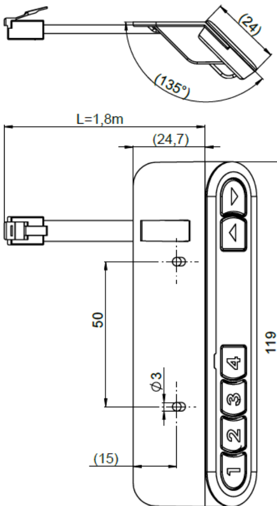
Abbildung 18: Abmaße des Memory Handschalters LD6LC
