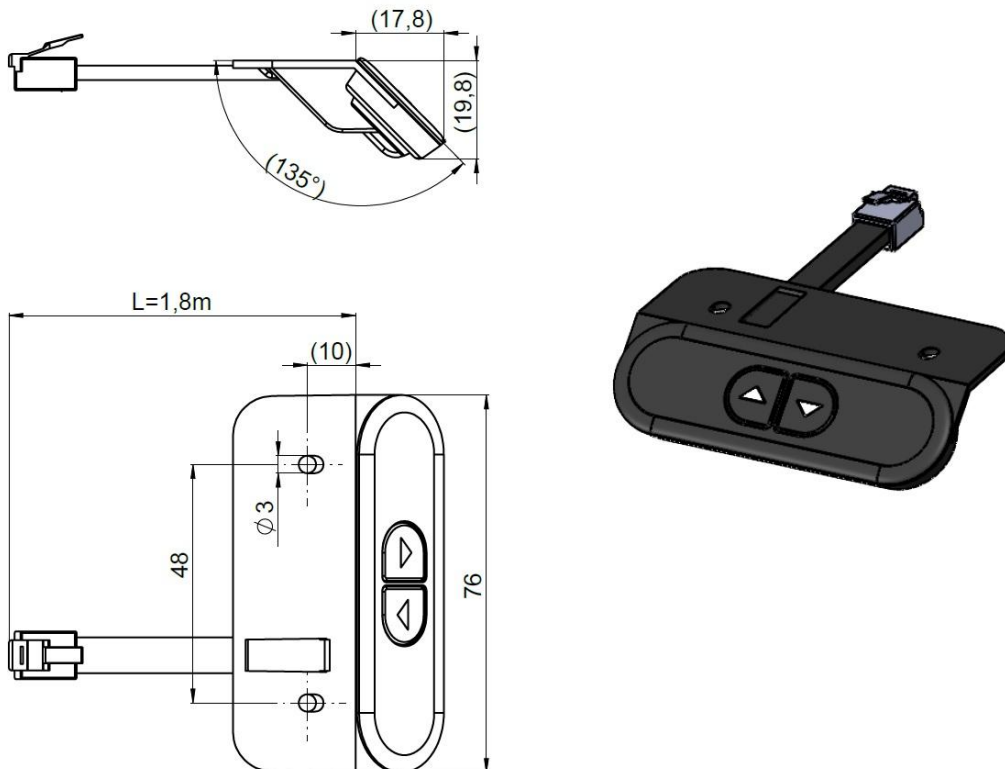
Abbildung 16: Abmaße UP / Down Handschalter LM2LCDP
