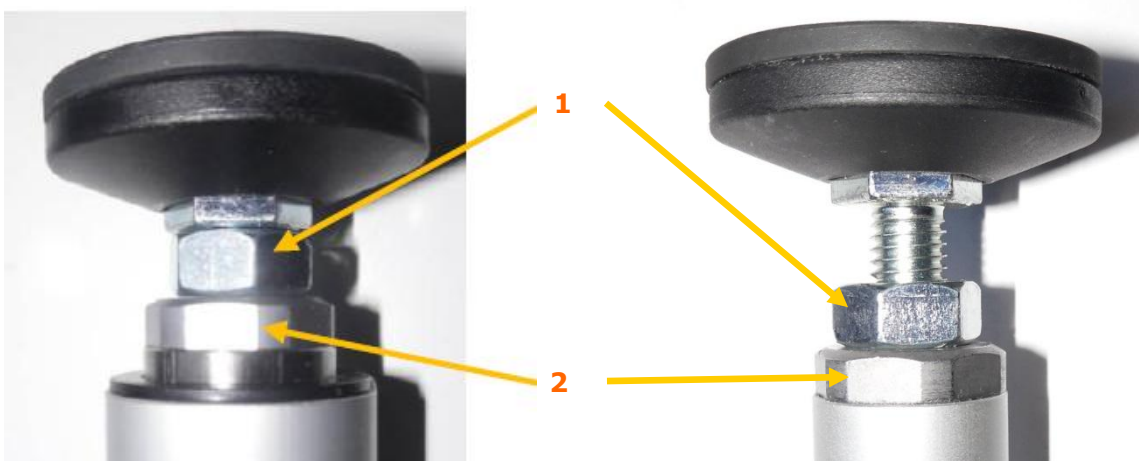
Abbildung 24: Verstellbarer Stellfuß (Optional)
