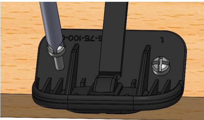
Abbildung 15: Befestigung UP / Down Handschalter LM2LCDP
