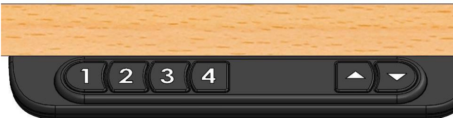
Abbildung 26: Memory Handschalter LD6LC (optional bzw. für mehr als ein 4 Bein System notwendig)
