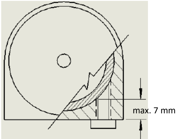
Abbildung 9: Maximale Schraubtiefe
